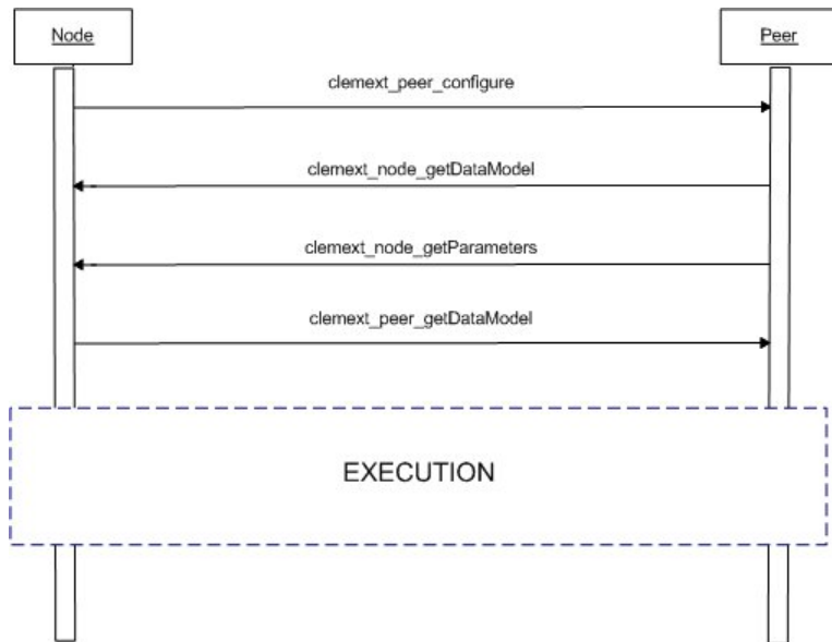
図 99. 一般的なピアとノードの相互作用のブロック
