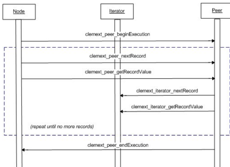
図 100. 一般的な実行ブロック
