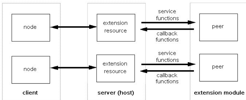
図 97. CLEF API アーキテクチャー
