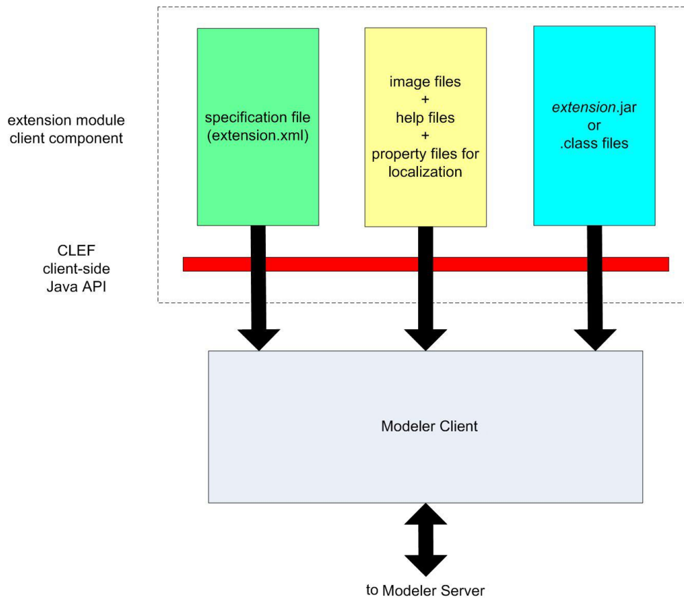
図 1. クライアント側コンポーネント
