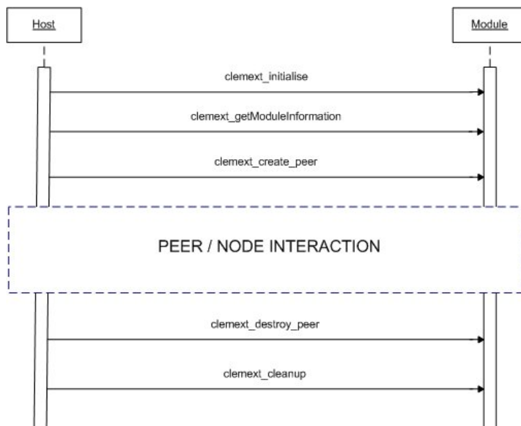
図 98. 一般的なプロセス・フロー
