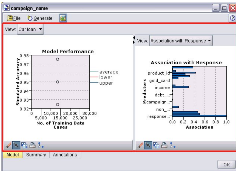
図 43. 拡張オブジェクト・パネルが強調表示されたモデル出力ウィンドウ
